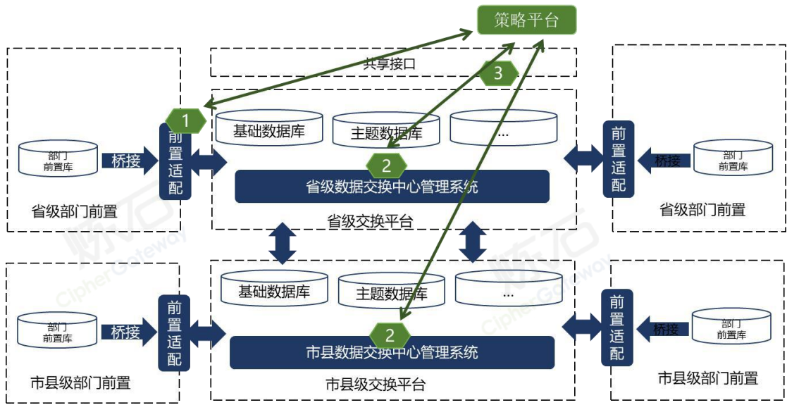
图 27 建设政务大数据交换共享平台安全增强设计示意
