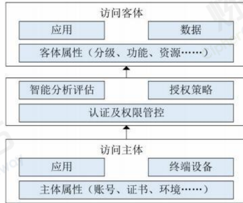
图 31 数据中台“零信任”安全防护架构
